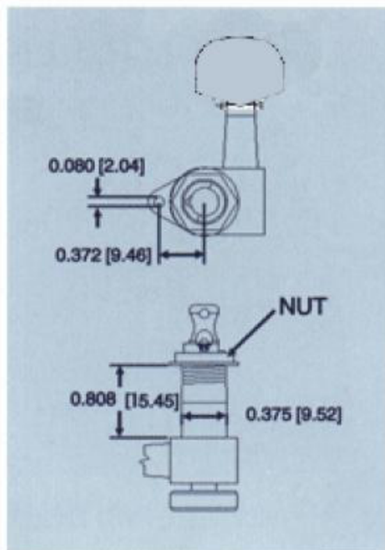
3+3 AUTO-TRIM DIMENSIONS
